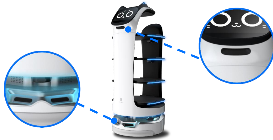
RGBD-Tiefenkamera
